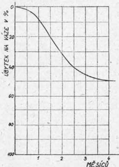
Rozklad smrkového dřeva houbou Poria Vaillantii (D. C.). Fr. Osa X: doba v měsících, po kterou houba působí, osa Y: postupující rozklad dřeva vyjádřený v % úbytku na váze.
